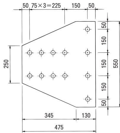
● H 300型 H 350型 t=12\text{mm} (20kg)
