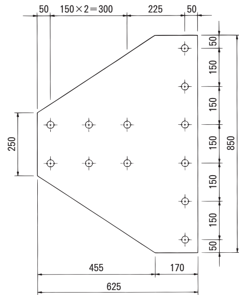
● H 400型 t=16\text{mm} (50kg)
