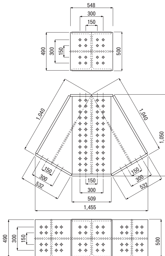
● H500型 火打ブロック30° (910kg)
