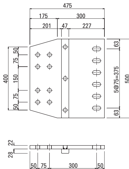
● H 500型 t=16\text{mm} (45kg)
